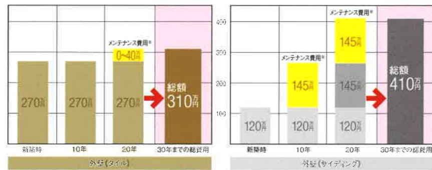
ライフサイクルコスト(LCC)のシミュレーション
